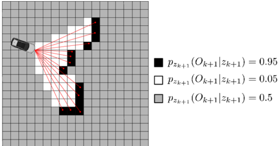
Şekil 4.5 2B Izgara Doluluk Haritası [14]
