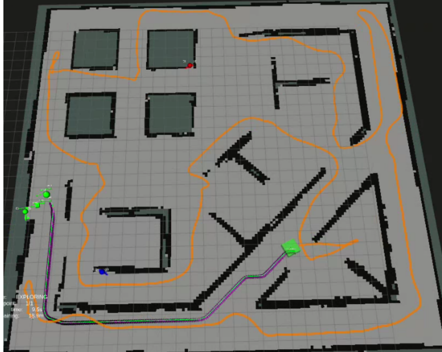
Şekil 5.3 Complex Office Keşif Yolu
