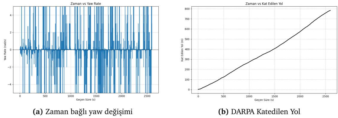
Şekil 5.15 DARPA Parkurunda Hareket Analizi
