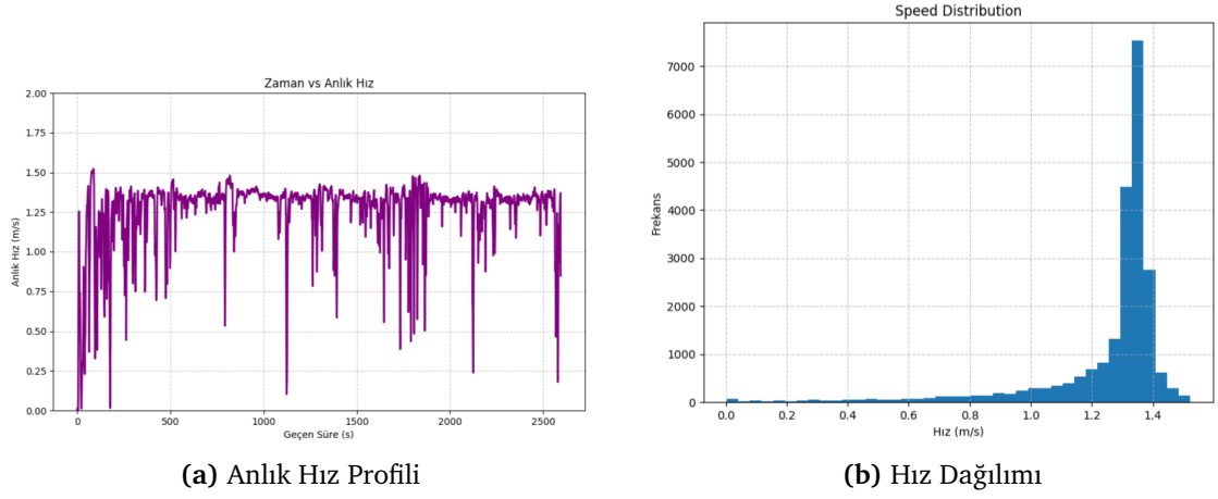
Şekil 5.14 DARPA Parkurunda Hız Analizi
