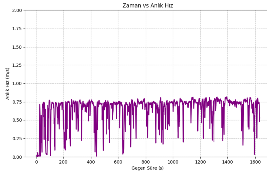
(a) Anlık Hız Profili
