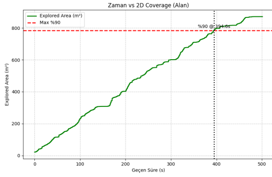
(a) 2B Alan Kapsaması
