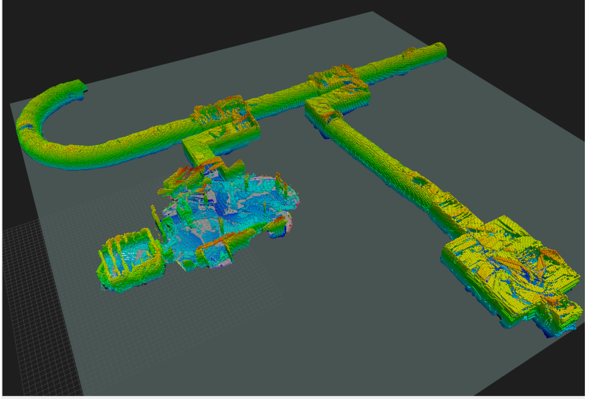
Şekil 5.12 Darpa 3B Octomap Haritası
