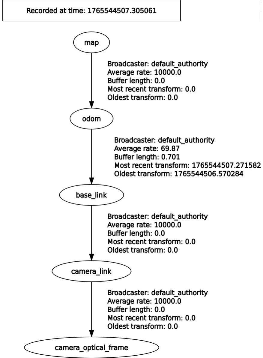
Şekil 4.9 ROS TF ağacı
