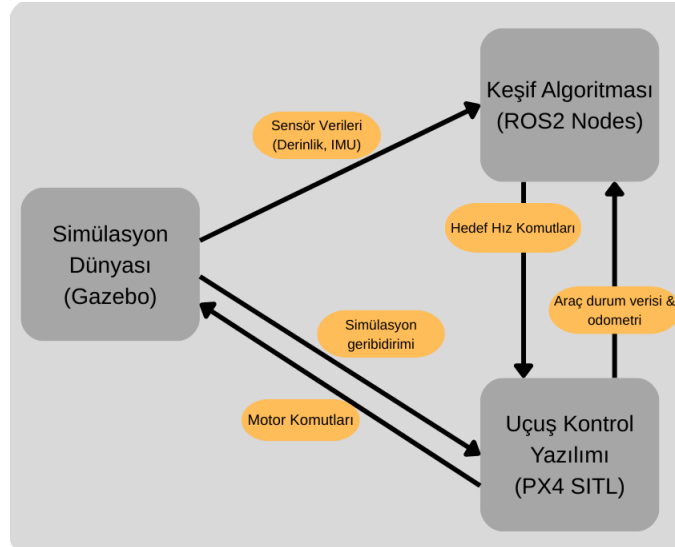
Şekil 3.1 Sistem Mimarisi
